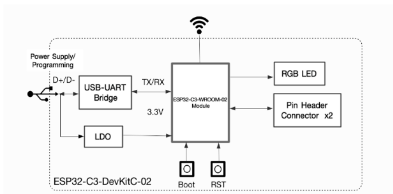
Ilustración 3 Diagrama ESP 32
