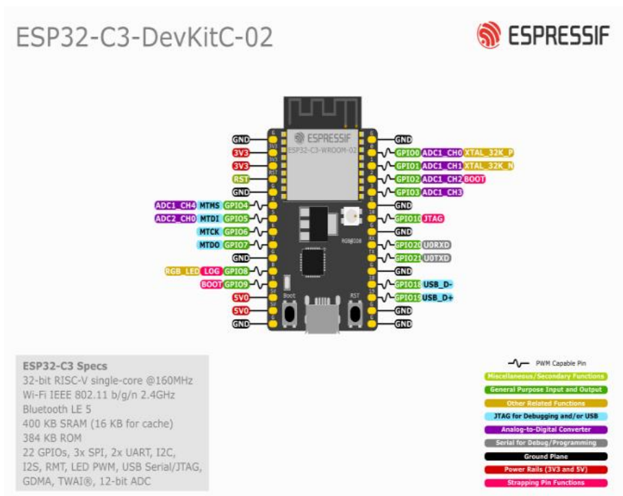
Ilustración 4 Pinout
